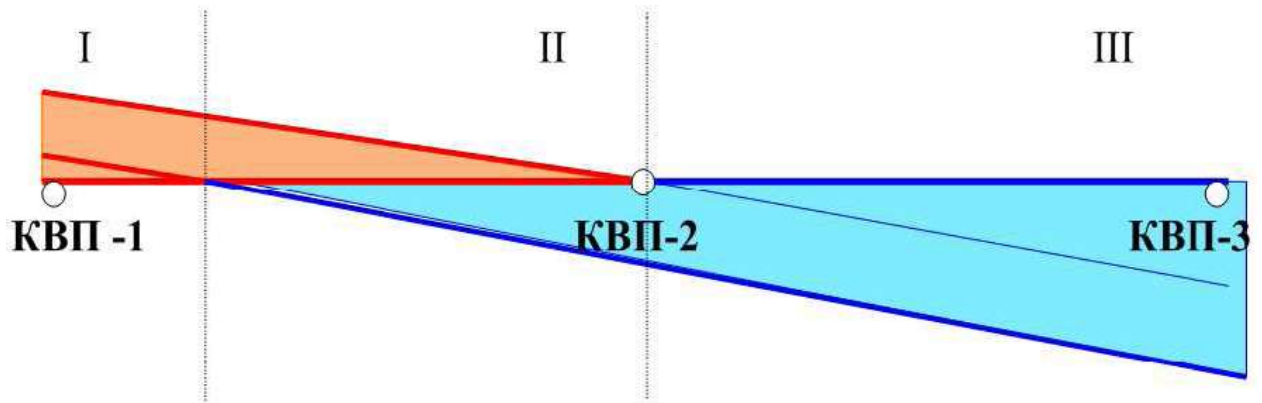
Рис. 1. Діаграма зсуву потенціалів на ділянці газопроводу: I – анодна зона; II – знаковмінна зона; III – катодна зона (зона захисту)
