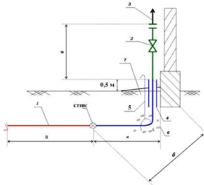
Рис.1. Структура газопроводу-вводу:
